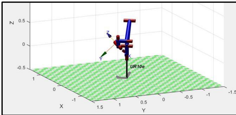
Fig. 18 – Singularidad (q_3, q_4)_1
