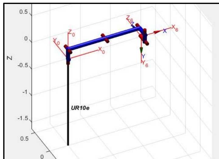
Fig. 14 – Posición cero con offset nulo
