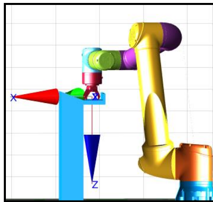
Fig. 27 – Colocación de la tapa en la mesa
