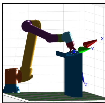
Fig. 25 – Punto de agarre de la tapa y extracción de la pastilla
