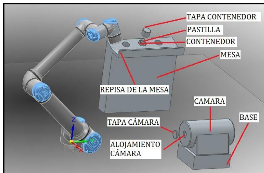
Fig. 1 – Modelo 3D de la celda de trabajo
