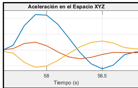
Fig. 33 – Zoom sobre aceleración cartesiana
