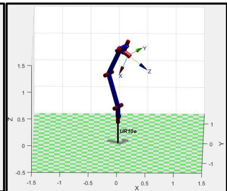
Figura 19 – Singularidad (q_3, q_4)_2
