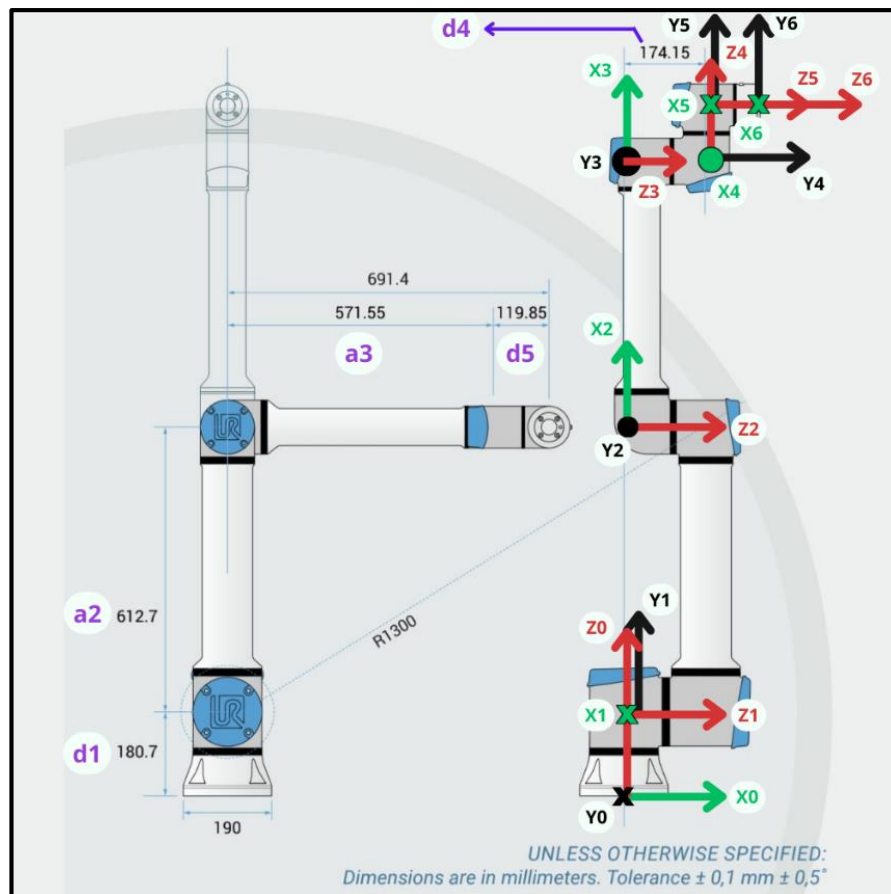
Fig. 13 – Aplicación de la convención de Denavit-Hartenberg
